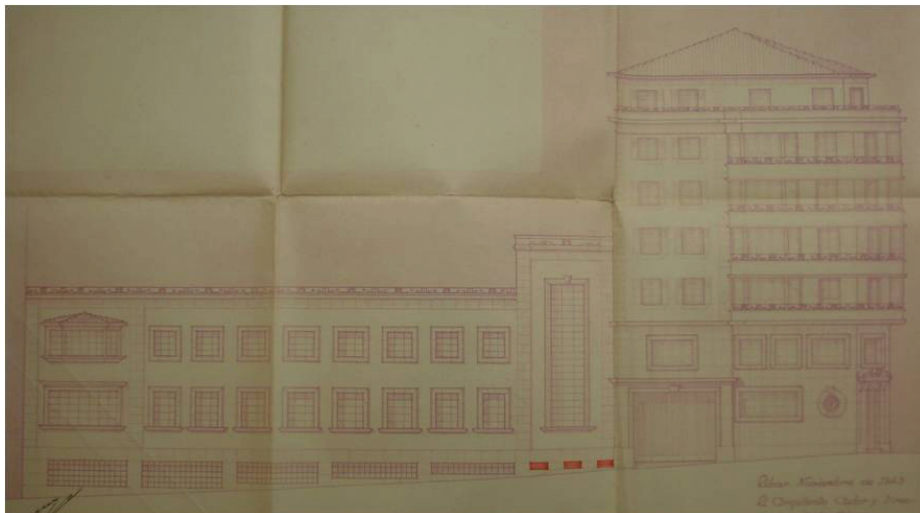
112. irudia. Arragueta kaleko tailerra eta etxea. Izen bereko kaleko plano. Raimundo Alberdi, Eibarren 1943ko azaroan. Eibarko Udal Artxiboa. Udal Funtza. Sig. 6861.72.
