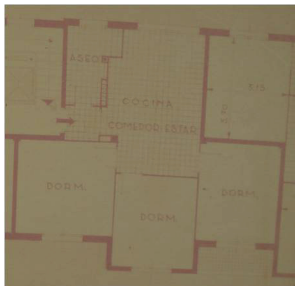
92. irudia. Ipuruako udal-etxebizitzaren oinplanoa (xehetasuna). Joaquín Domínguez Elósegui, Donostia 1952ko apirila.. Eibarko Udal Artxiboa. Udal Funtsa. Sig. 3.162.
